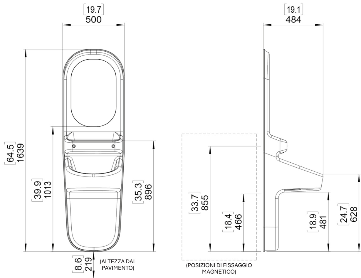
Lavabo Arc (Accessibile)
